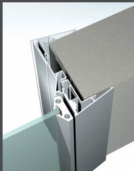
Particolare stipite Detail of the doorjamb Détail du montant Detail des Pfostens Detalle de la jamba
