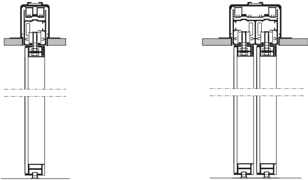
Applicazione su cartongesso con binario a 1, 2 vie incassato a filo del soffitto | Application on plasterboard with 1, 2 way built-in ceiling rail | Application sur placoplâtre avec rail 1, 2 voies au plafond encaissé | Anwendung auf Gipskartonplatten mit 1,2 Wege eingelassene Deckenschiene | Aplicación al pladur con el binario de 1, 2 vías a ras del techo
