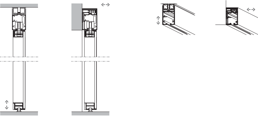
Il carrello consente la regolazione verticale del pannello scorrevole | The truck allows vertical adjustments of the sliding panel | Le chariot permet le réglage vertical du panneau coulissant | Der Wagen ermöglicht eine vertikale Einstellung der Schiebetür | El carrito permite el ajuste vertical del panel corredero
