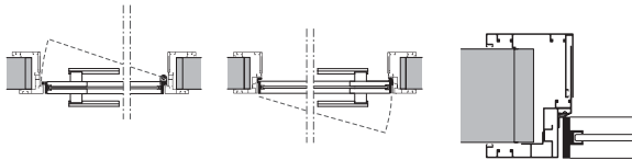
Stipiti a 45° | Jams 45° | Montants à 45° | Türstockverkleidung 45 ° | Jambas en 45°
