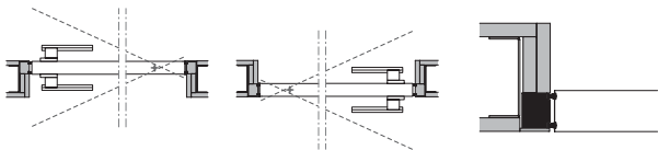
Filomuro | Flush door | Ras de mur | Drehtüren zum Ziehen | Enrasada a la pared
