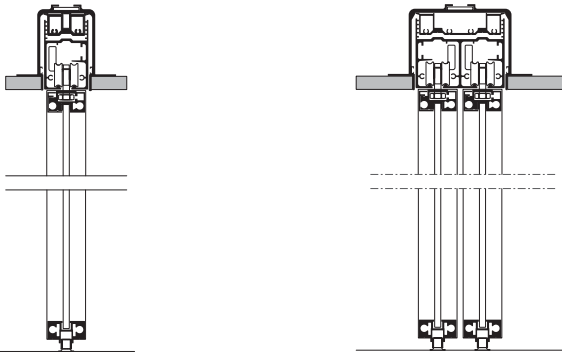
Applicazione su cartongesso con binario a 1, 2 vie incassato a filo del soffitto | Application on plasterboard with 1, 2 way built-in ceiling rail | Application sur placoplâtre avec rail 1, 2 voies au plafond encaissé | Anwendung auf Gipskartonplatten mit 1,2 Wege eingelassene Deckenschiene | Aplicación al pladur con el binario de 1, 2 vías a ras del techo
