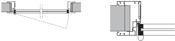
Stipiti a 45° | Jambas 45° | Montants à 45° | Türstockverkleidung 45 ° | Jambas en 45°
