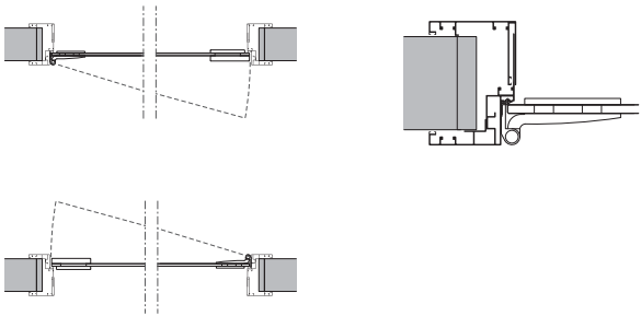
Stipiti a 45° | Jambas 45° | Montants à 45° | Türstockverkleidung 45 ° | Jambas en 45°
