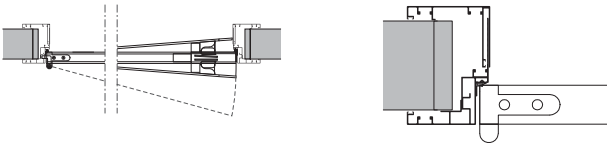
Stipiti a 45° | Jams 45° | Montants à 45° | Türstockverkleidung 45 ° | Jambas en 45°
